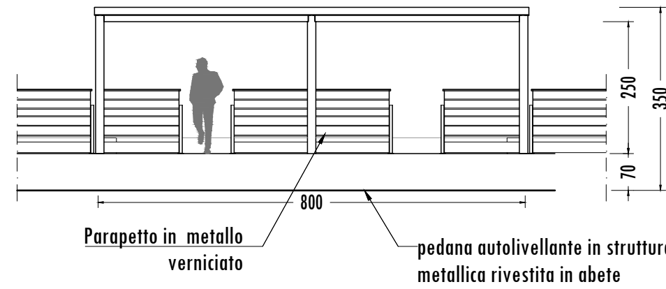
Prospetto posteriore 2 scala 1:100
