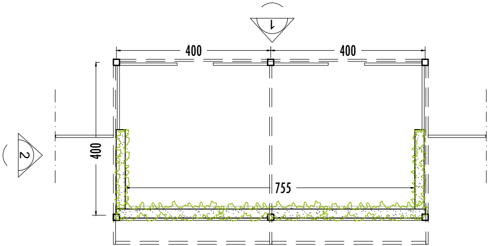
Pianta (1-A) scala 1:100
