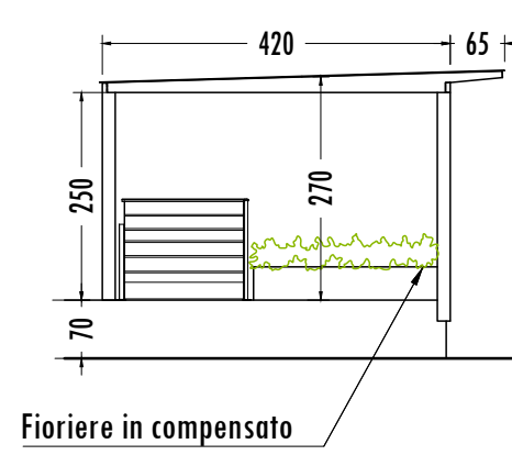
Prospetto laterale 1 scala 1:100
