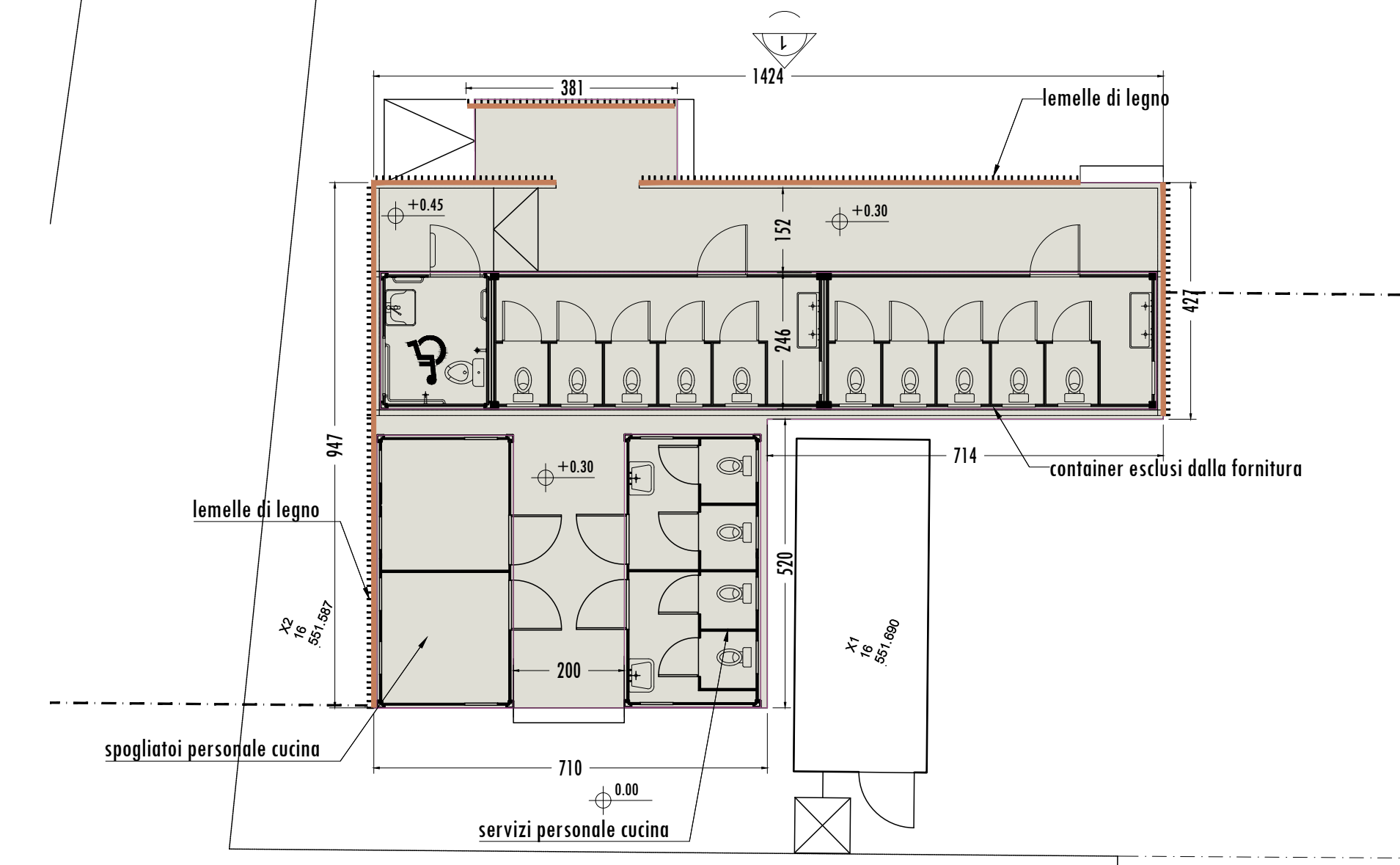
Planimetria scala 1:100
